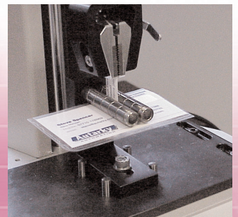
peel
